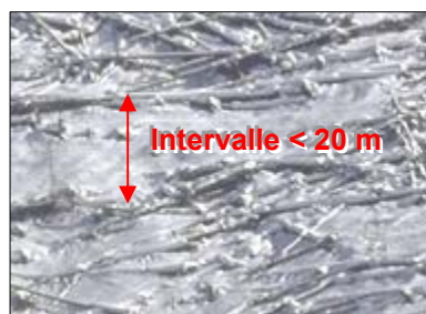
Figure 5: Intervalle maximal entre les éléments servant d'ouvrages paravalanches en raison de leur hauteur d'action (surface laissée telle quelle à Disentis lors des avalanches de l'hiver 1998–1999).
