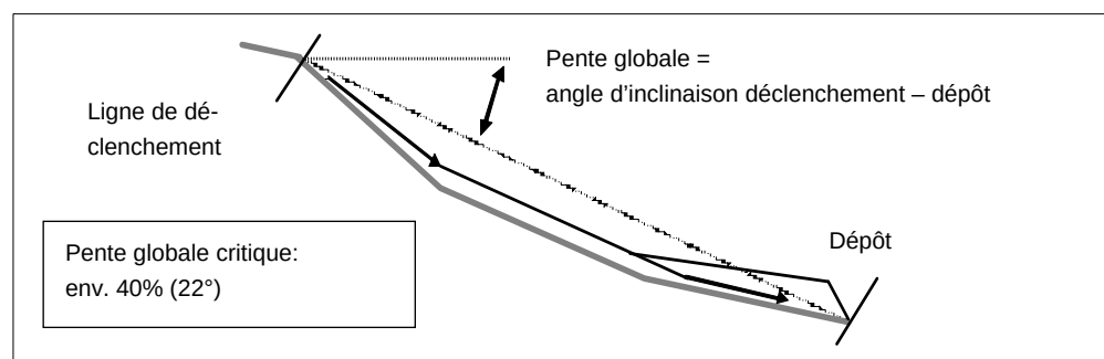
Figure 3: Définition de la pente globale; figure de TEUFEN (1993), légèrement modifiée.
