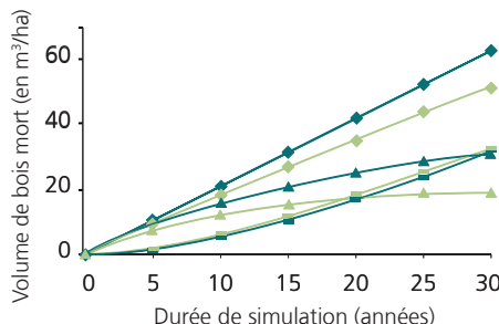
Fig. 7. Modélisation de l'accumulation de bois mort pendant 30 ans pour des peuplements inexplotés d'épicéas et de hêtres, le bois mort sur pied se distinguant de celui au sol. Hypothèses pour les peuplements initiaux dans le perchis (à gauche): volume de bois = 180 \text{ m}^3/\text{ha} (épicéa) et 220 \text{ m}^3/\text{ha} (hêtre). DHP de la tige de surface terrière moyenne = 15 \text{ cm} . Hypothèses concernant la futaie (à droite): volume de bois = 500 \text{ m}^3/\text{ha} (épicéa) et 400 \text{ m}^3/\text{ha} (hêtre). DHP de la tige de surface terrière moyenne = 35 \text{ cm} (épicéa) et 30 \text{ cm} (hêtre). Ces deux peuplements ne comportent à l'origine aucun bois mort.
