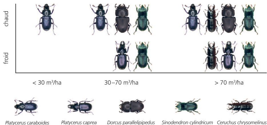
Fig. 10. Les représentants de la famille des lucanes (Lucanidae) sont de bons indicateurs de la quantité de bois mort et de la température dans les hêtraies (LACHAT et al. 2012).
