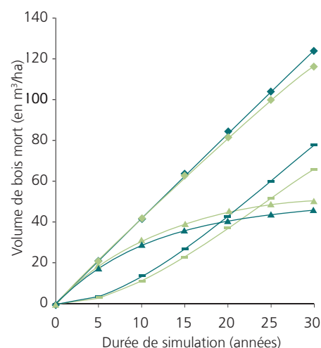
Fig. 7. Modélisation de l'accumulation de bois mort pendant 30 ans pour des peuplements inexplotés d'épicéas et de hêtres, le bois mort sur pied se distinguant de celui au sol. Hypothèses pour les peuplements initiaux dans le perchis (à gauche): volume de bois = 180 \text{ m}^3/\text{ha} (épicéa) et 220 \text{ m}^3/\text{ha} (hêtre). DHP de la tige de surface terrière moyenne = 15 \text{ cm} . Hypothèses concernant la futaie (à droite): volume de bois = 500 \text{ m}^3/\text{ha} (épicéa) et 400 \text{ m}^3/\text{ha} (hêtre). DHP de la tige de surface terrière moyenne = 35 \text{ cm} (épicéa) et 30 \text{ cm} (hêtre). Ces deux peuplements ne comportent à l'origine aucun bois mort.
